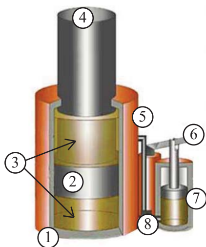
5-rasm. Yuk ko'tarish moslamasi (domkrat): 1 – asos; 2 – porshen; 3 – ishchi suyuqlik (jidkost); 4 – tayanch nuqtasi; 5 – silindr; 6 – dasta; 7 – nasos; 8 – bosimni pasaytiruvchi klapan.
