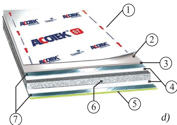
d – po'lat asosli: 1 – himoya plyonkasi, 2 – emal, 3 – grunt, 4 – termopolimer yelimi, 5 – himoya qoplamasi, 6 – innovatsion kompozit materiallar (alcotek), 7 – po'lat listlar.
