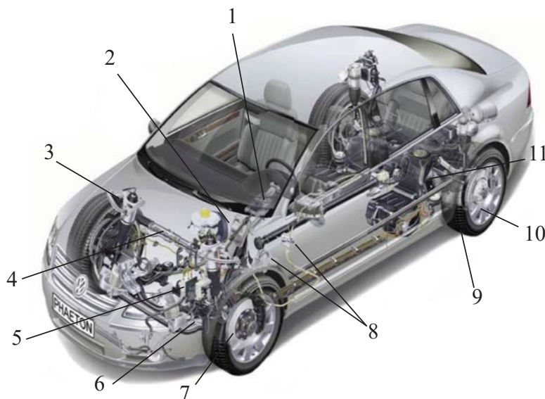
2-rasm, a. Yengil avtomobil konstruksiyasi: 1 – avtomatik boshqariladigan rul; 2 – tormoz kuchaytirish moslamasi; 3 – amortizatorlar; 4 – boshqarish uskunalar; 5 – piyodalarga qarshi ogohlantiruvchi tormoz tizimi; 6 – oldingi most (ko'prik); 7 – disk tormozi supporti birikmasi; 8 – tormoz pedali; 9 – shinalar; 10 – qotishma g'ildiraklar; 11 – orqa most (ko'prik).
