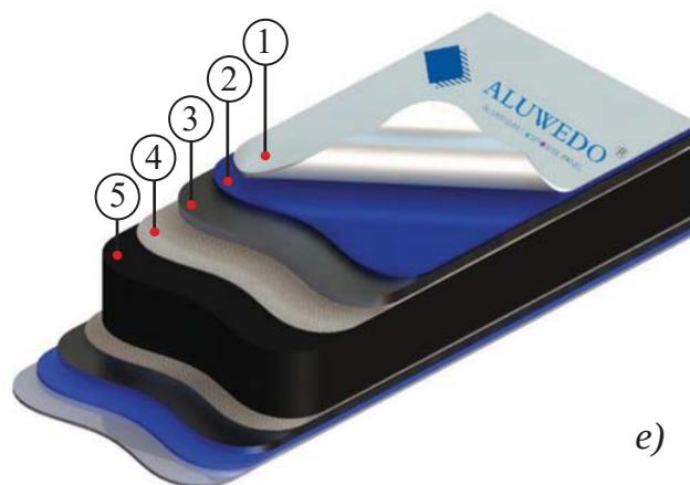
e – polimer asosli: 1 – himoya plyonkasi, 2 – bo'yoq bilan qoplangan qismi, 3 – aluminiy qatlam, 4 – yopishqoq qatlam, 5 – polietilen.
