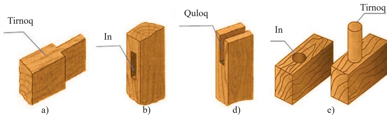
40-rasm. Duradgorlik birikmalarini hosil qilish elementlari.
